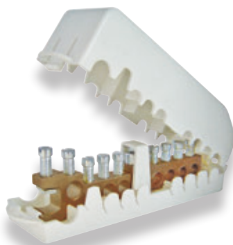
Répartiteur de terre 8 dérivation (Q130)
